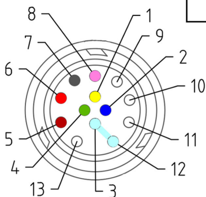
Schéma de câblage 13 BROCHES ( PRA06324 - PRA06334 )
