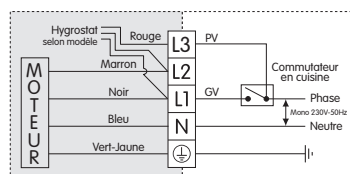
Schéma de câblage avec interrupteur
