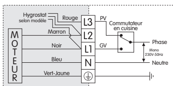
Schéma de câblage avec inverseur
