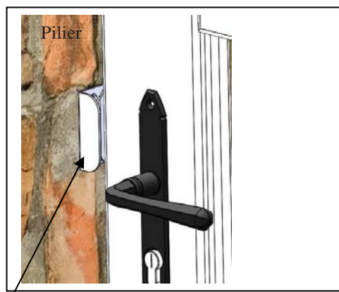
Gâche de réception
