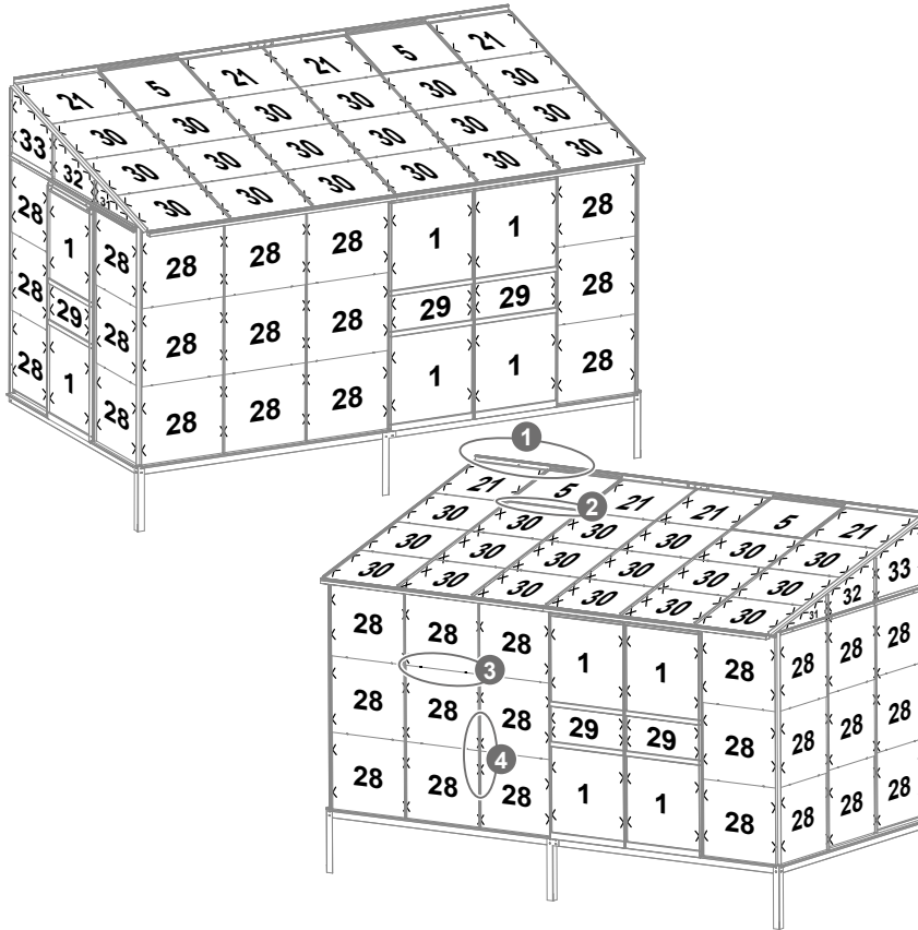
Pose de la lucarne sur faîtière par glissement. Anbringung des Fensters auf First durch Gleiten. Installing the window on roof ridge through sliding.
