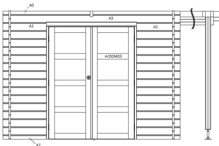
VOORZIJDE - FACADE
