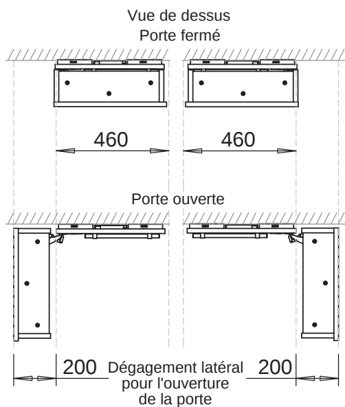
Porte à gauche
