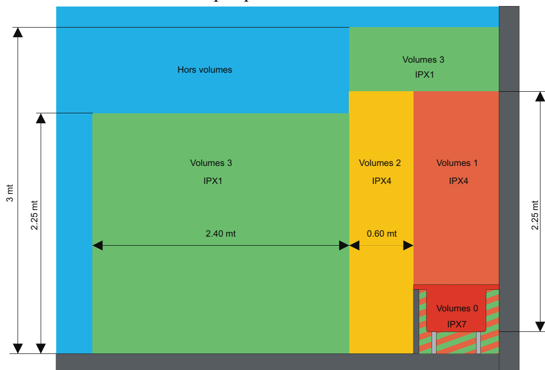
Graphique NFC 15-100
