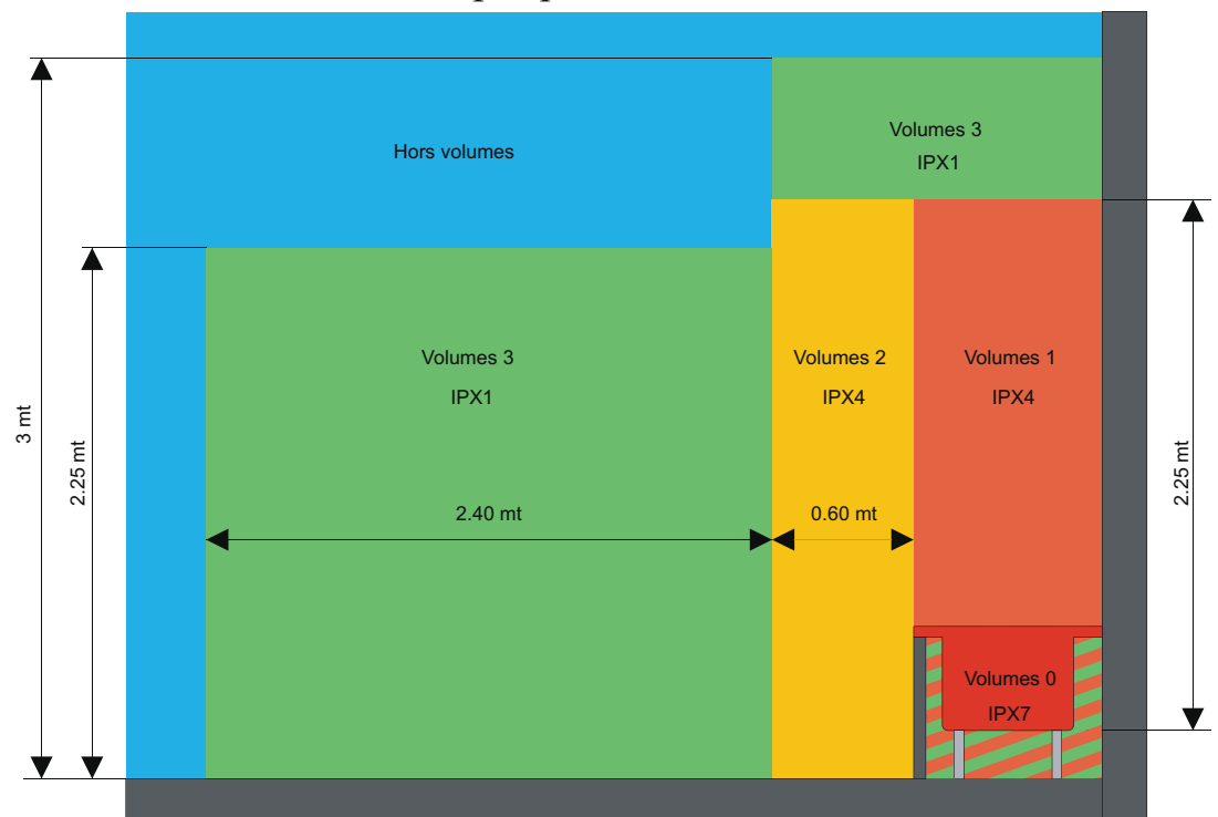
Graphique NFC 15-100
