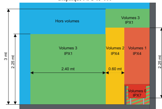
Graphique NFC 15-100
