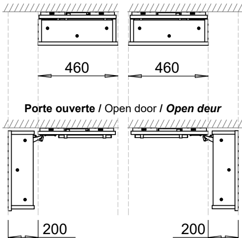
Dégagement latéral pour l'ouverture de la porte / Lateral clearance for door opening / Zijdelingse ruimte voor deuropening
