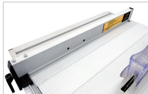
Guide parallèle traversant à double fixations Traversing parallel guide with double fixings
