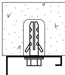
MUR DE BÉTON
