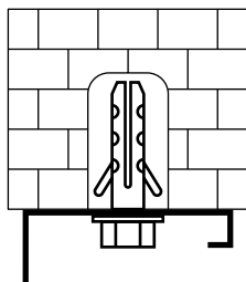
MUR DE BRIQUE
