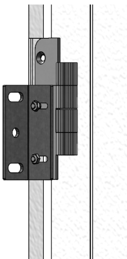
Position sur le vantail gauche
