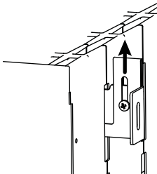
Support déverrouillé
