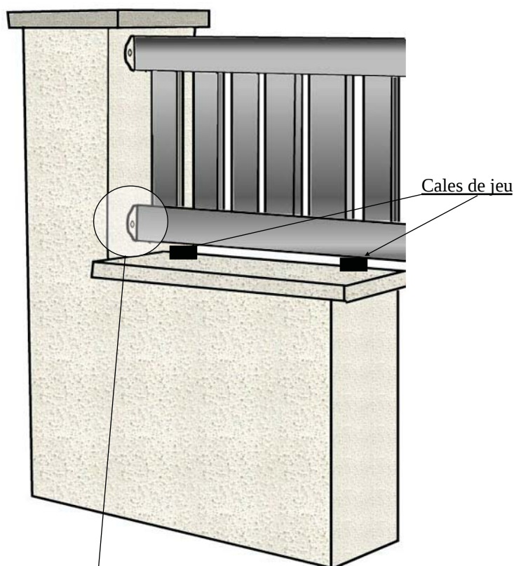
Fixation Alu 6
