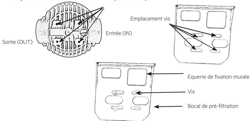
Schéma de montage
