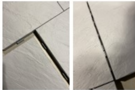
2 Centrer les clips en face des encoches et coller les dalles ou lames le plus possible avant clippage
