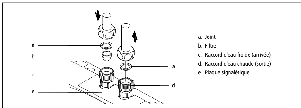
Fig. 6: « Raccordement des conduites d'eau »
