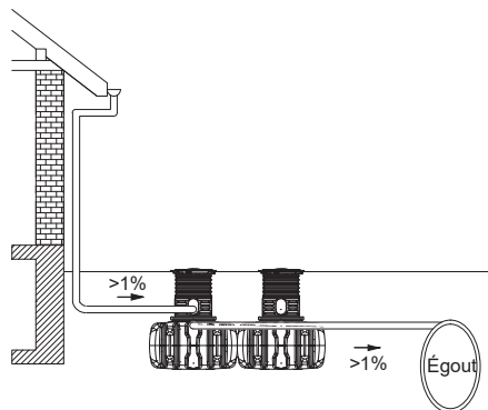
Fig. 31 : Schéma de raccordement – Exemple FLAT
