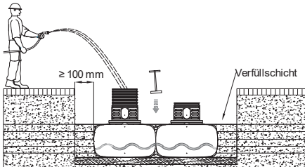
Abb. 27: Einsetzen und Verfüllen – FLAT
