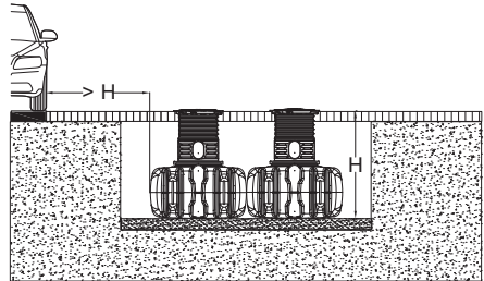
Fig.21: Distancia a las zonas de tráfico – ejemplo FLAT
