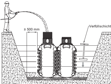
Abb. 29: Einsetzen und Verfüllen – MODULARIS
