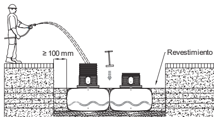
Fig.27: Inserción y relleno – FLAT
