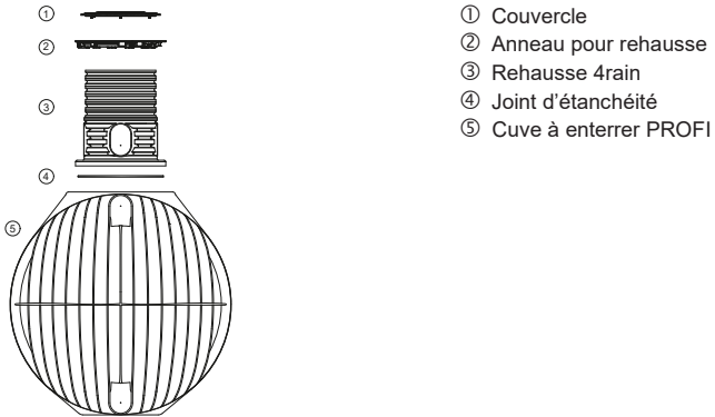
Fig. 17 : Composants – PROFi
