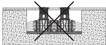
Fig.3: Aguas subterráneas/estratificadas – ejemplo FLAT
