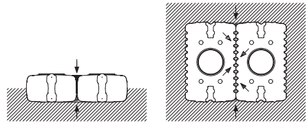
Fig. 28 : Cavités entre les cuves – FLAT
