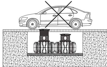
Abb. 2: Verkehrsbelastung – Beispiel FLAT
