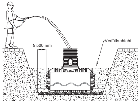
Abb. 30: Einsetzen und Verfüllen – COMPACT, PROFI
