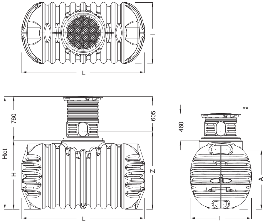
Fig. 8 : Dimensions – COMPACT
