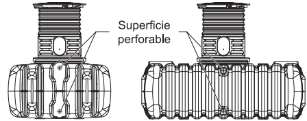
Fig.22: Superficies de perforación para conectar varios contenedores – FLAT
