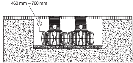
Fig. 1 : Hauteurs de recouvrement – Exemple FLAT
