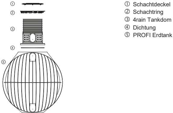
Abb. 17: Komponenten – PROFI
