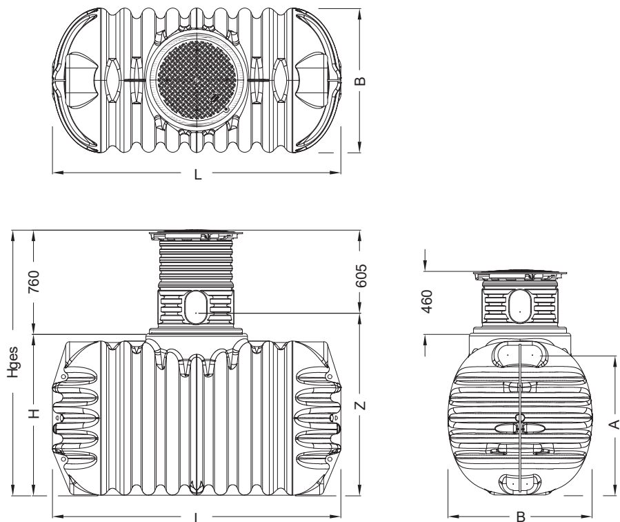
Abb. 8: Abmessungen – COMPACT
