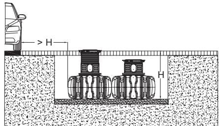
Abb. 21: Abstand zu Verkehrsflächen – Beispiel FLAT
