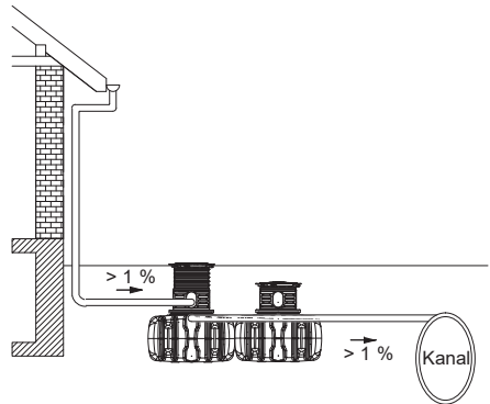
Abb. 31: Anschluss-Schema – Beispiel FLAT
