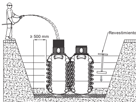
Fig.29: Inserción y relleno – MODULARIS
