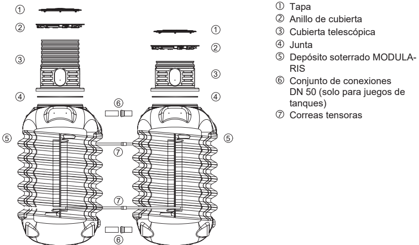
Fig. 15: Componentes – MODULARIS
