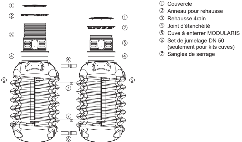
Fig. 15 : Composants – MODULARIS
