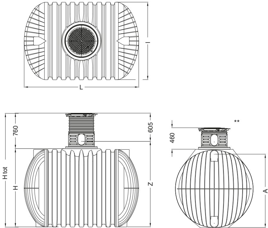
Fig. 9 : Dimensions – PROFI
