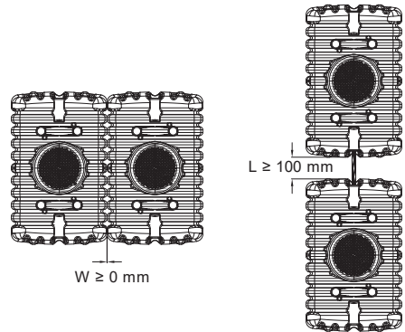
Fig.23: Conexión de varios contenedores – FLAT
