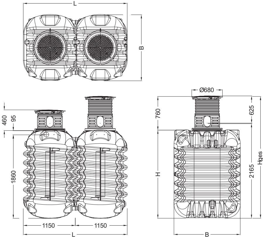
Abb. 7: Abmessungen – MODULARIS
