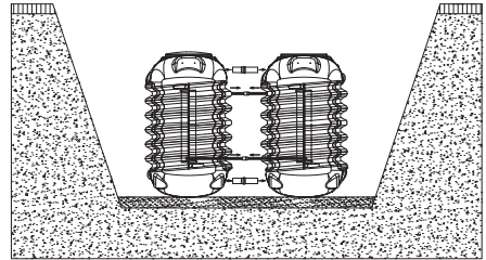
Fig. 24 : Jumelage de plusieurs cuves – MODULARIS
