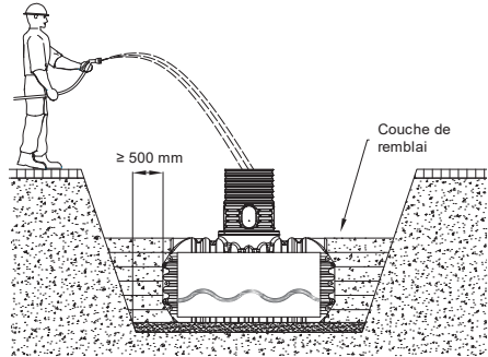
Fig. 30 : Mise en place et remplissage – COMPACT, PROFI
