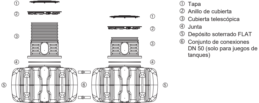
Fig.10: Componentes – FLAT
