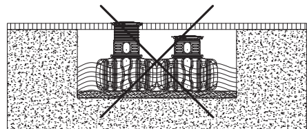
Abb. 3: Grund-/Schichtenwasser – Beispiel FLAT
