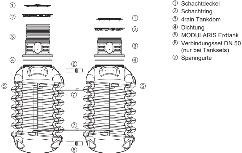
Abb. 15: Komponenten – MODULARIS
