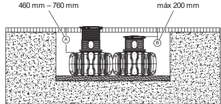
Fig.1: Alturas de cobertura – ejemplo FLAT
