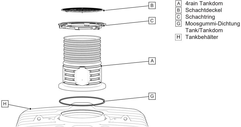
Abb. 33: Tankdom und Abdeckung – Montageübersicht
