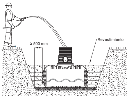
Fig.30: Inserción y relleno – COMPACT, PROFI
