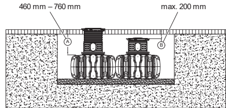
Abb. 1: Überdeckungshöhen – Beispiel FLAT
