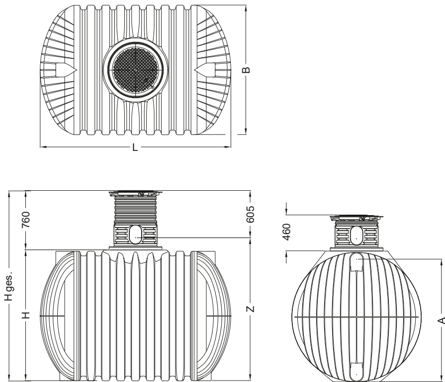
Abb. 9: Abmessungen – PROFI
