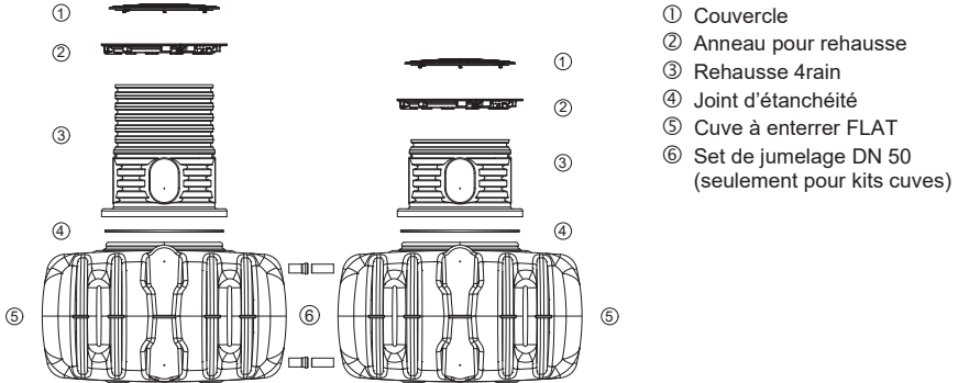
Fig. 10 : Composants – FLAT
