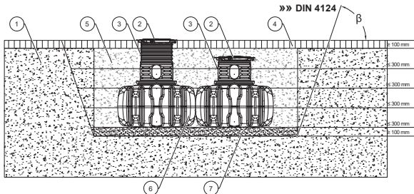
Abb. 18: Einbauschema – Beispiel FLAT
