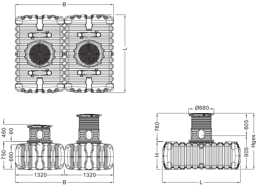
Abb. 4: Abmessungen – FLAT S
