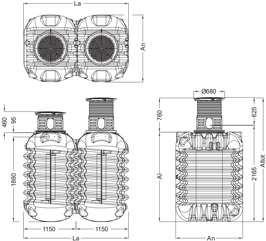
Fig.7: Dimensiones – MODULARIS
