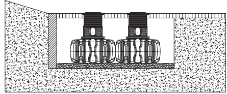
Fig. 19 : Installation sur terrain en pente – Exemple FLAT
