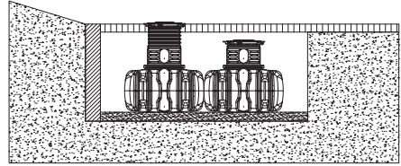
Abb. 19: Einbau in Hanglage – Beispiel FLAT
