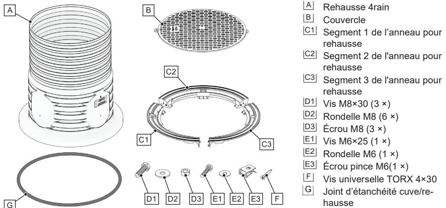
Fig. 32 : Rehausse 4rain et couvercle – Vue éclatée
