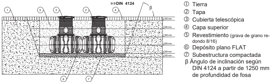
Fig.18: Esquema de instalación – ejemplo FLAT
