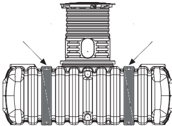
Abb. 11: Schnittdarstellung Stützrohre – FLAT S/M
