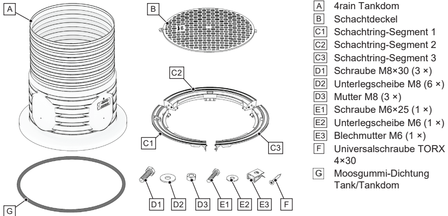
Abb. 32: Tankdom und Abdeckung – Teileübersicht
