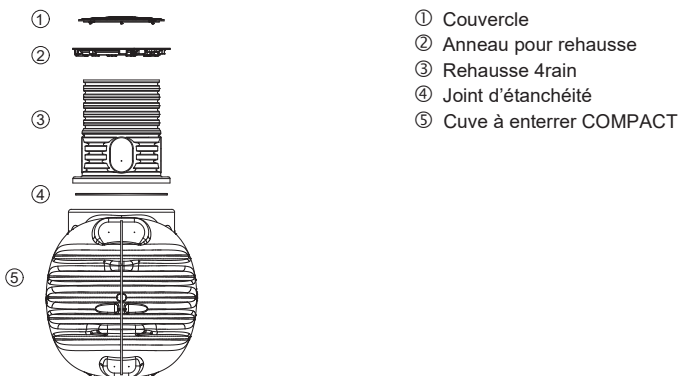
Fig. 16 : Composants – COMPACT
