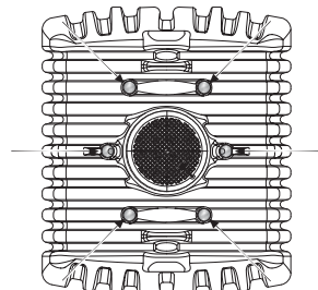
Fig.14: Vista general / Posiciones de los tubos de soporte – FLAT L
