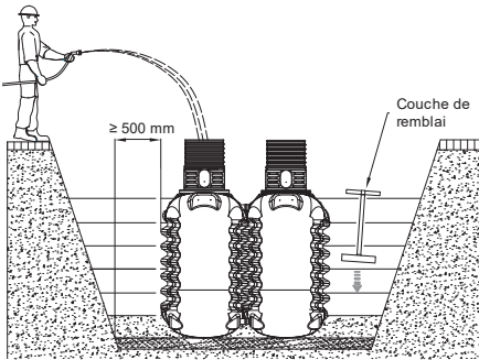
Fig. 29 : Mise en place et remplissage– MODULARIS
