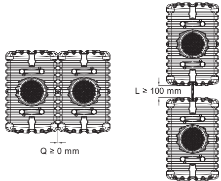
Abb. 23: Verbinden mehrerer Behälter – FLAT
