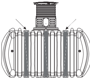
Fig.13: Vista en sección de los tubos de soporte – FLAT L
