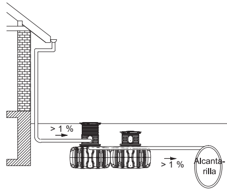
Fig.31: Esquema de conexión – ejemplo FLAT
