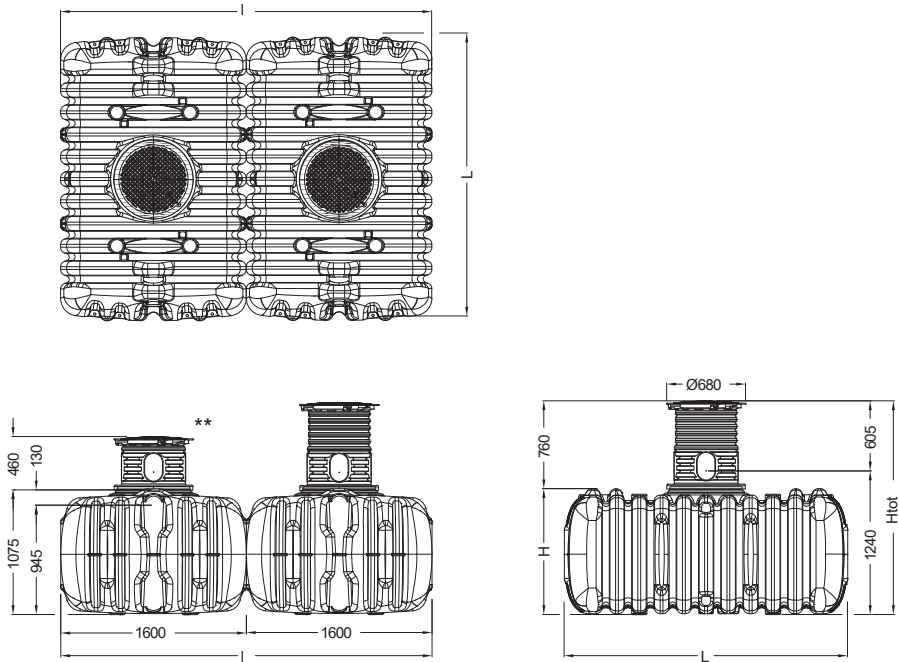
Fig. 5 : Dimensions – FLAT M
