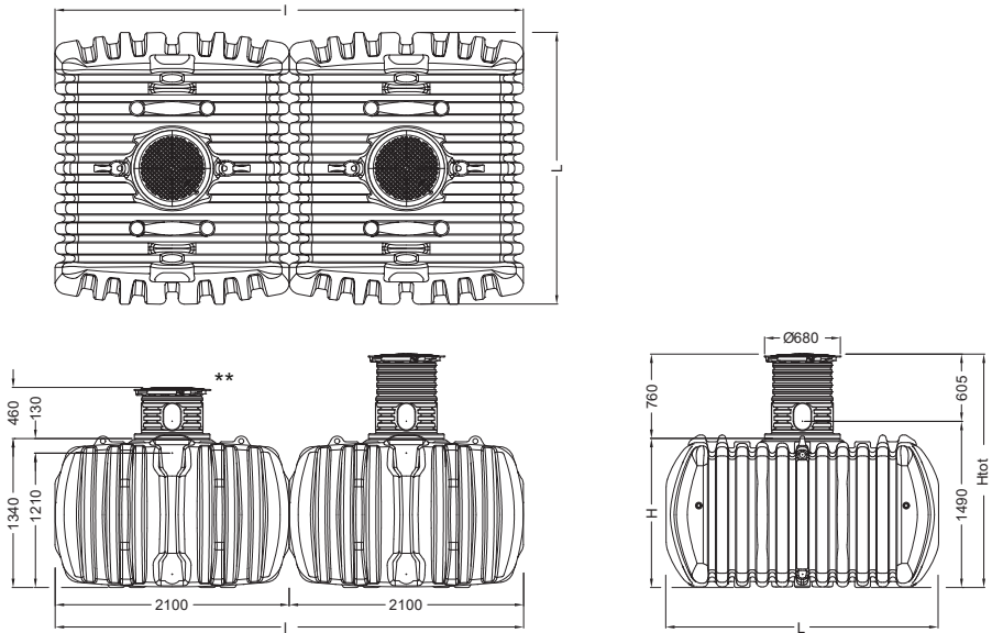
Fig. 6 : Dimensions – FLAT L
