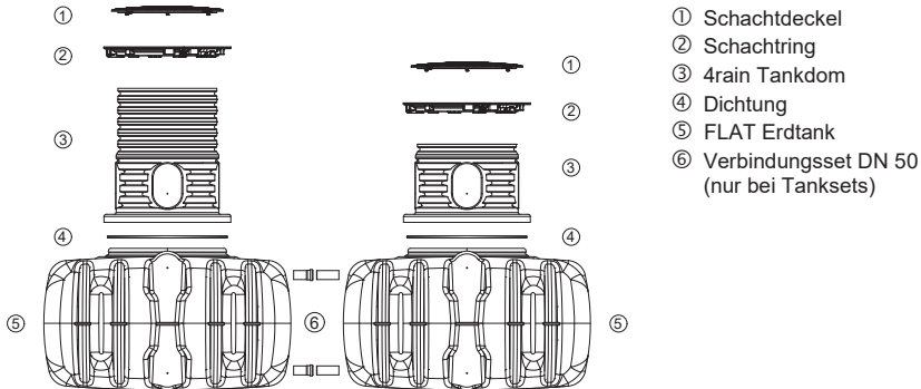
Abb. 10: Komponenten – FLAT
