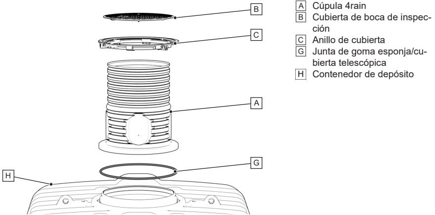
Fig. 33: Cúpula y tapa – Vista general del montaje
