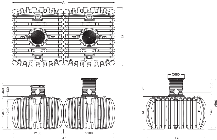
Fig. 6: Dimensiones – FLAT L
