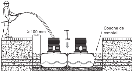
Fig. 27 : Mise en place et remplissage– FLAT
