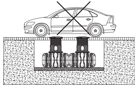
Fig.2: Carga de tráfico – ejemplo FLAT
