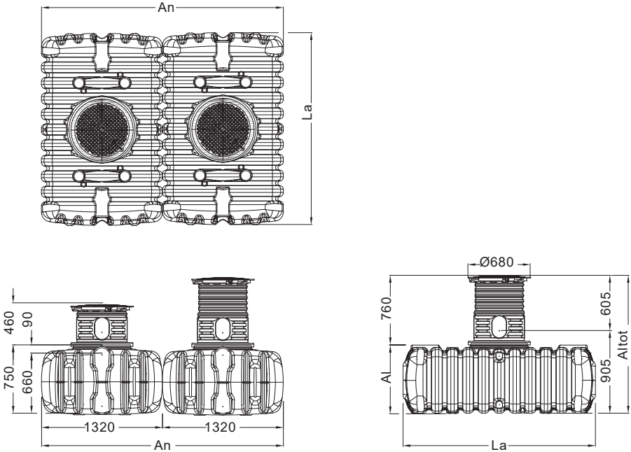
Fig.4: Dimensiones – FLAT S
