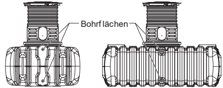
Abb. 22: Bohrflächen zum Verbinden mehrerer Behälter – FLAT
