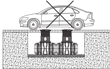
Fig. 2 : Charge de circulation – Exemple FLAT
