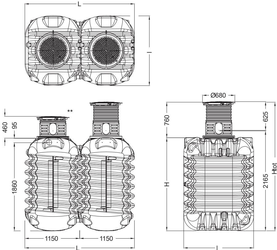
Fig. 7 : Dimensions – MODULARIS
