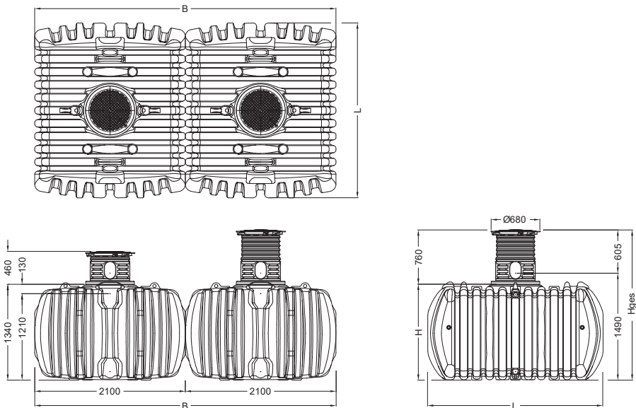
Abb. 6: Abmessungen – FLAT L
