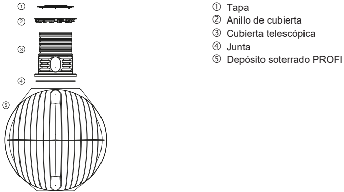
Fig. 17: Componentes – PROFÍ
