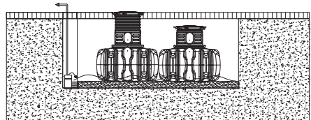
Abb. 20: Einbau bei Wasser in der Baugrube – Beispiel FLAT
