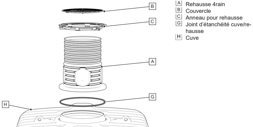
Fig. 33 : Rehausse 4rain et couvercle – Aperçu du montage
