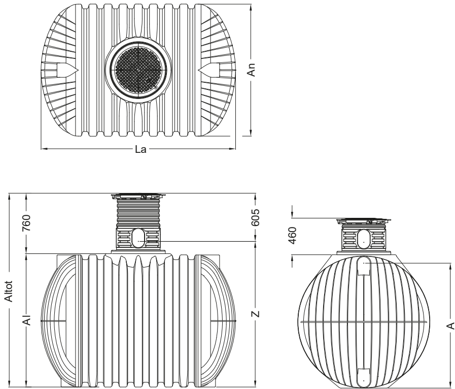
Fig. 9: Dimensiones – PROFÍ
