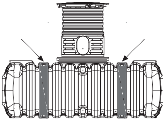
Fig.11: Vista en sección de los tubos de soporte – FLAT S/M
