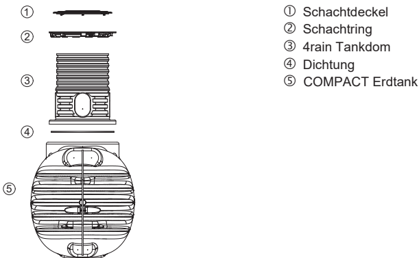
Abb. 16: Komponenten – COMPACT
