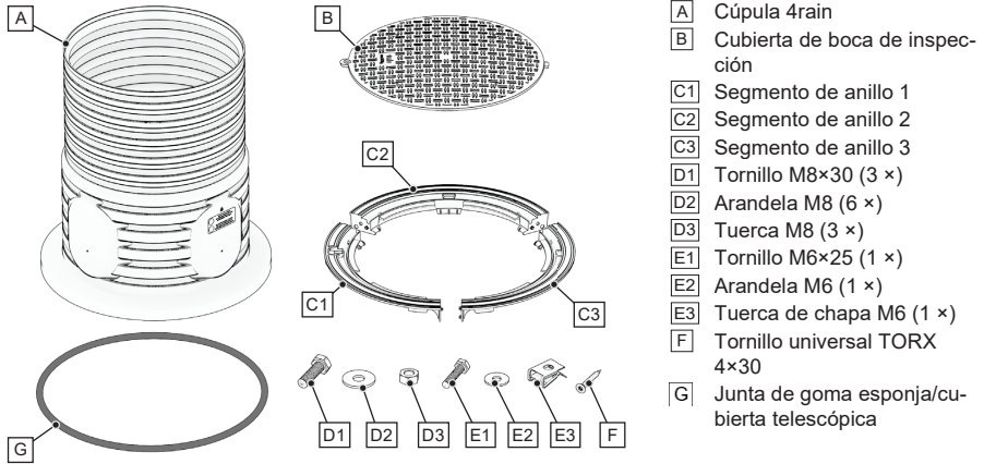
Fig. 32: Cúpula y tapa – Vista general de las piezas
