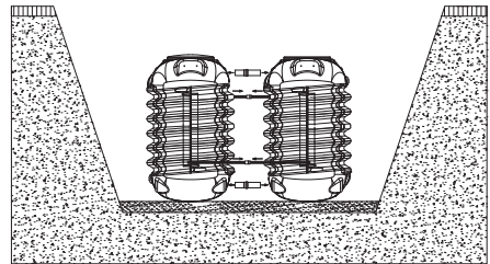
Fig.24: Conexión de varios contenedores – MODULARIS
