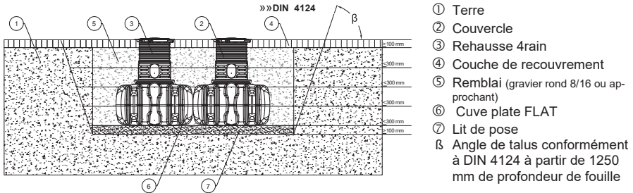
Fig. 18 : Schéma d'installation – Exemple FLAT
