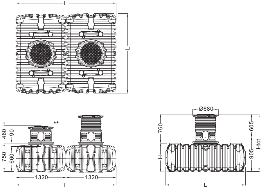
Fig. 4 : Dimensions – FLAT S
