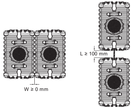
Fig. 23 : Jumelage de plusieurs cuves – FLAT
