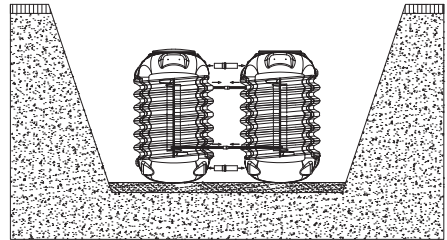
Abb. 24: Verbinden mehrerer Behälter – MODULARIS
