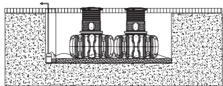
Fig.20: Instalación con agua en la fosa de excavación – ejemplo FLAT
