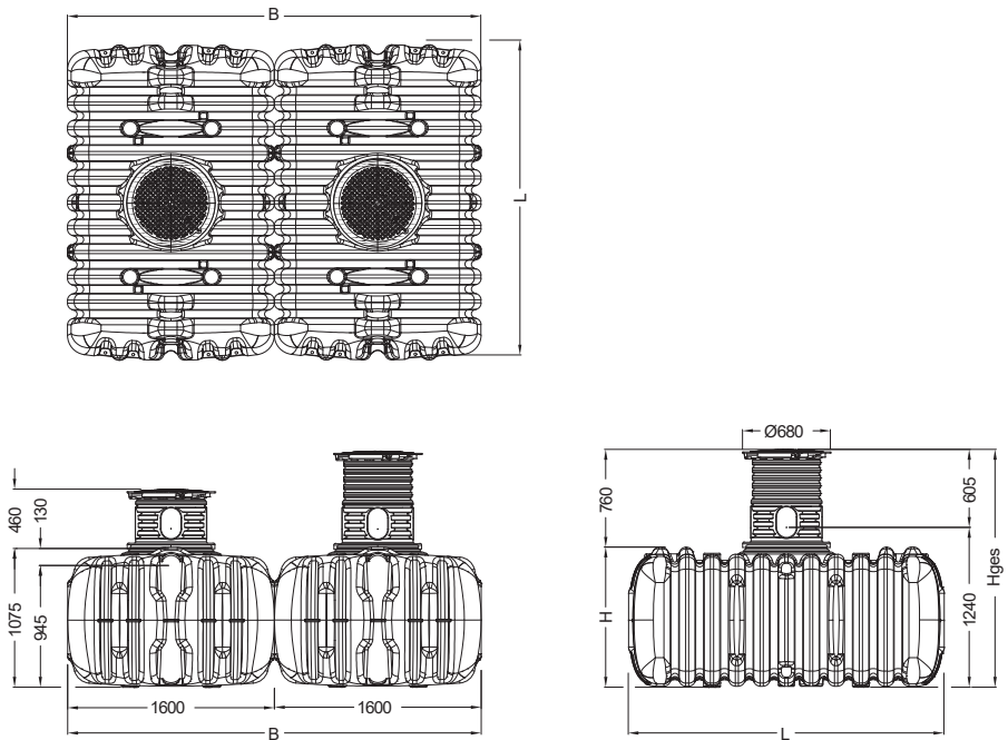
Abb. 5: Abmessungen – FLAT M
