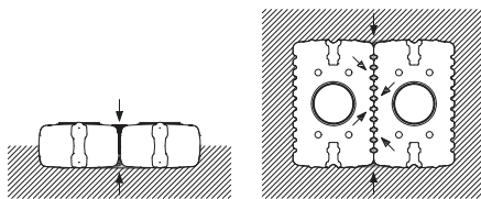
Fig.28: Cavidades entre contenedores – FLAT
