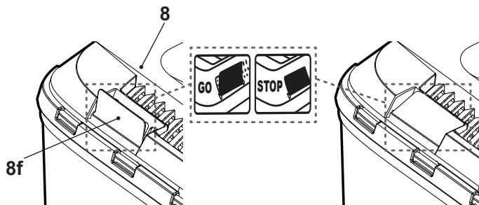
Illustration 13 position ouverte
