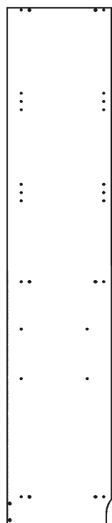
T. x1 2200 x 404 x 16 mm
