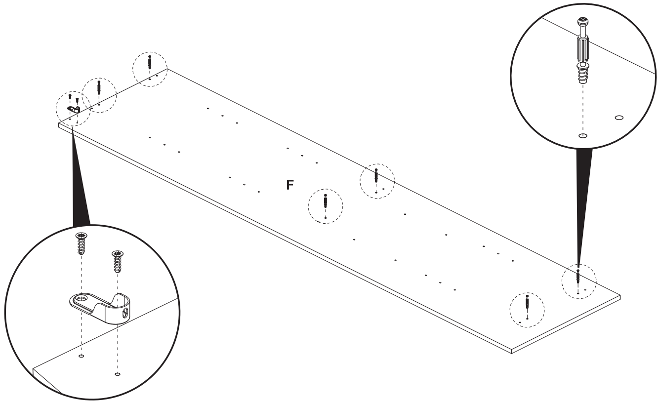
1. x1 (18 x 45,5 x 12 mm)
