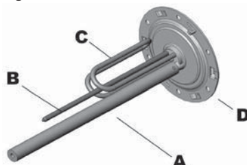
Figure 1 - Résistance thermoplongée + anode en magnésium
