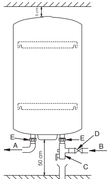
Figure 6 - Cotes d'installation
