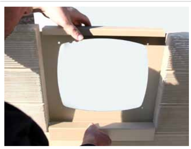
Mise en place de la plaque pour fixation du skimfiltre.
