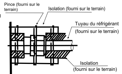
Procédure d'isolation de la tuyauterie
