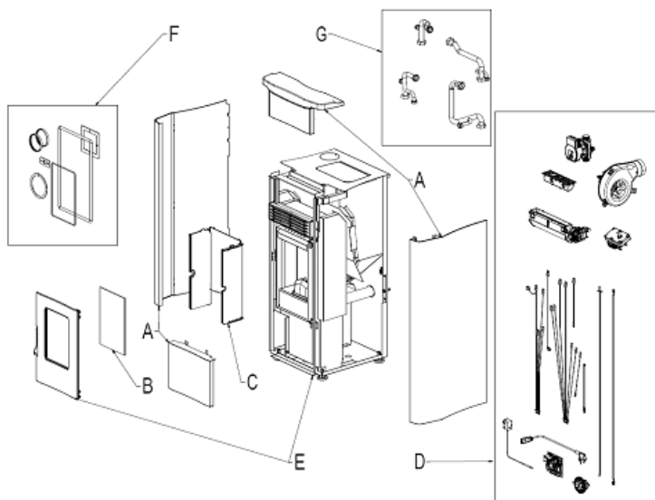
Fig. 1 - Dessin éclaté
