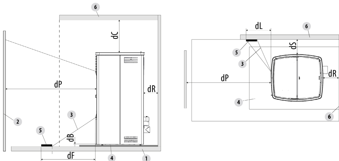
Fig. 18 - Distances de sécurité
