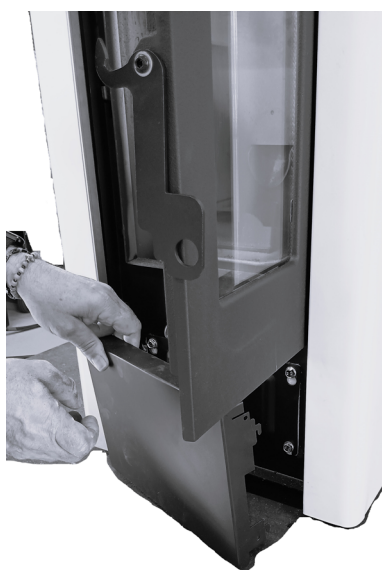
Fig. 34 - Décrochage du cache frontal
