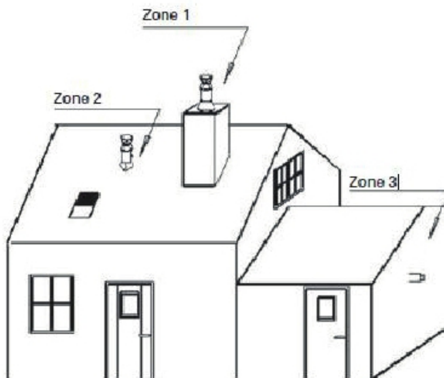
Fig. 10 - Definition des zones d'implantation
