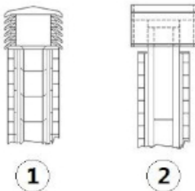
Fig. 6 - Sortie de toit coupe-vent
