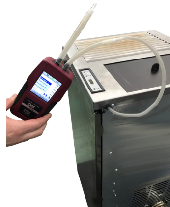
Fig. 29 - Connexion du pressostat numérique 1
