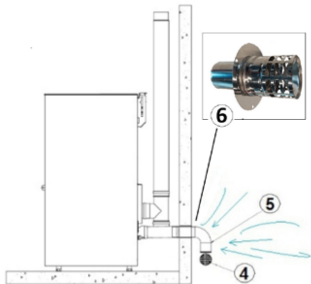
Fig. 9 - Prise d'air pour installation en chambre étanche
