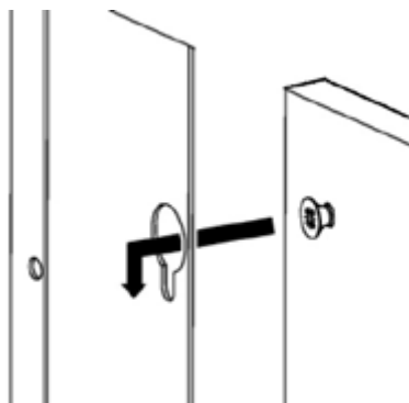
Fig. 48 - Détail de l'accrochage
