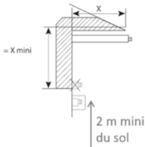
Fig. 14 - Rebord de toit
