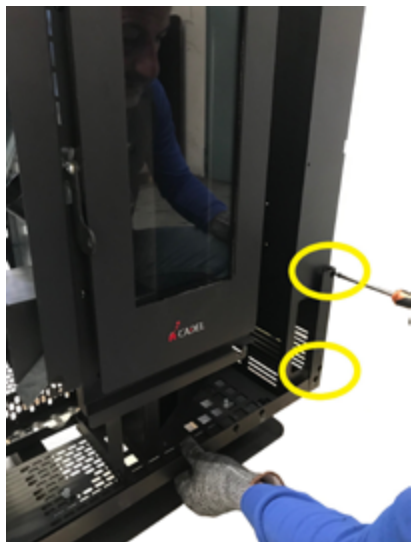
Fig. 50 - Fixation de l'étrier inférieur
