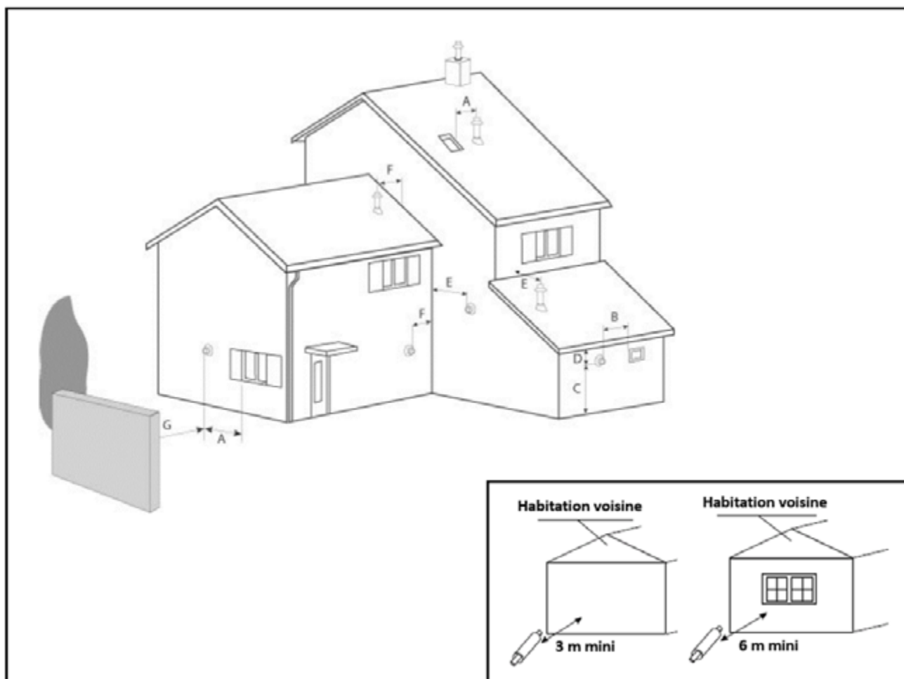
Fig. 13 - Position des terminaux
