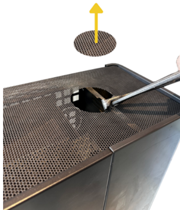
Fig. 79 - Casser la prédécoupe
