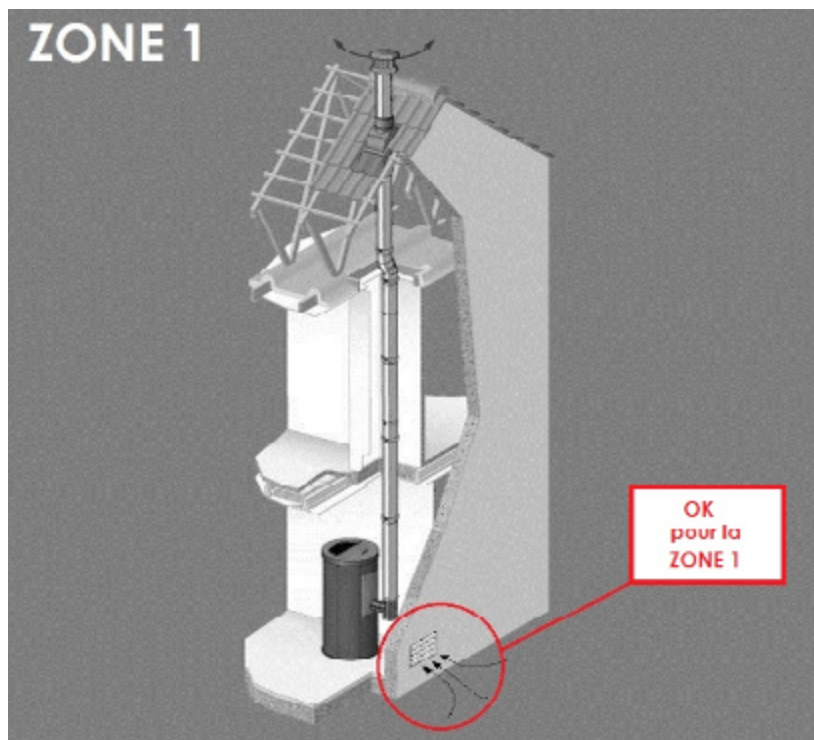
Fig. 15 - Installation possible pour tous les poêles (ZONE 1)
