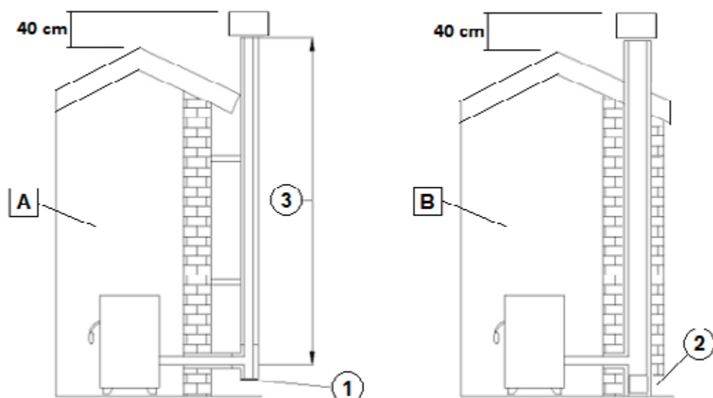
Fig. 3 - Conduit de fumées
