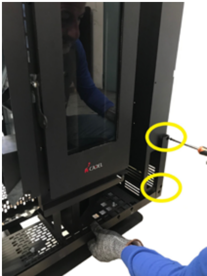
Fig. 43 - Fixation de l'étrier inférieur
