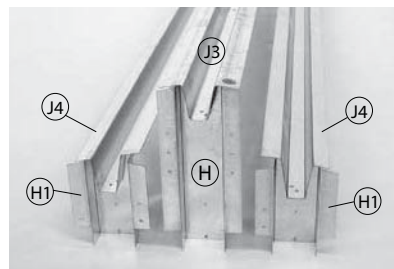
Nur Gr. 5 u. 7 / Sizes 5 and 7 only Taille 5 + 7 / Misura 5 + 7 Dachträger (J4) und Firststütze (H1) Roof beams (J4) and ridge supports (H1) porte-toit (J4) et support de faîtière (H1) trave tetto (J4) sostegno colmo (H1)
