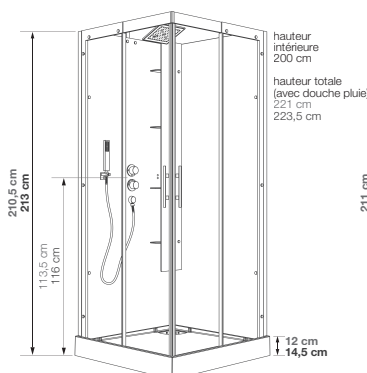
Cotes pour le modèle C80
