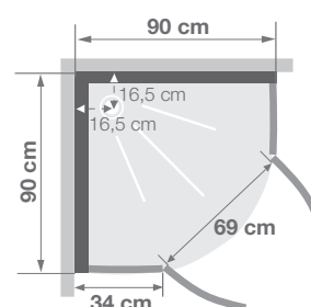
Horizon R90 - version thermostatique - couleur acier
