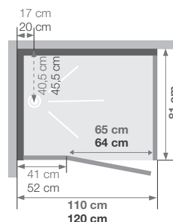
Horizon 120 x 91 - version hydro+hammam - couleur perle noire
