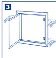
3 Poser le cadre, recourber les pattes de fixation et visser le cadre dans la cloison.
