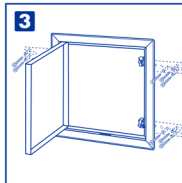
3 Poser le cadre, recourber les pattes de fixation et visser le cadre dans la cloison.
