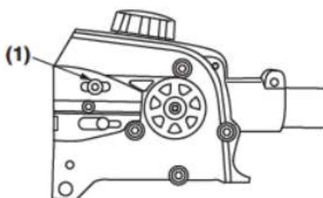
(1) Orifice d'huile
