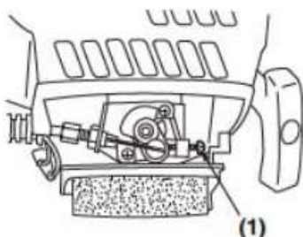
(1) Vis de réglage du ralenti
