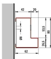
Détail cadre Tunnel(ref. MR1)
