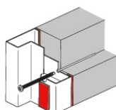
Détail d'installation cadre Tunnel(ref. MR1)
