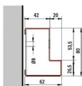
Détail cadre Tunnel(ref. MR1)
