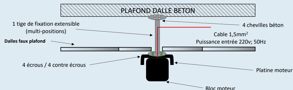
Tige télescopique & inclinable
