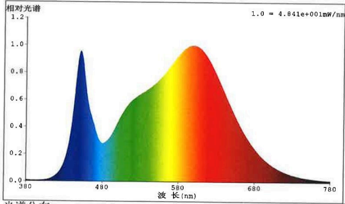
光谱分布
