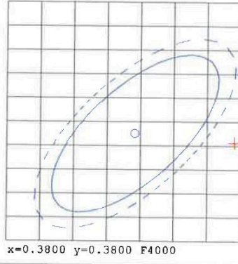
CIE1931色品图
