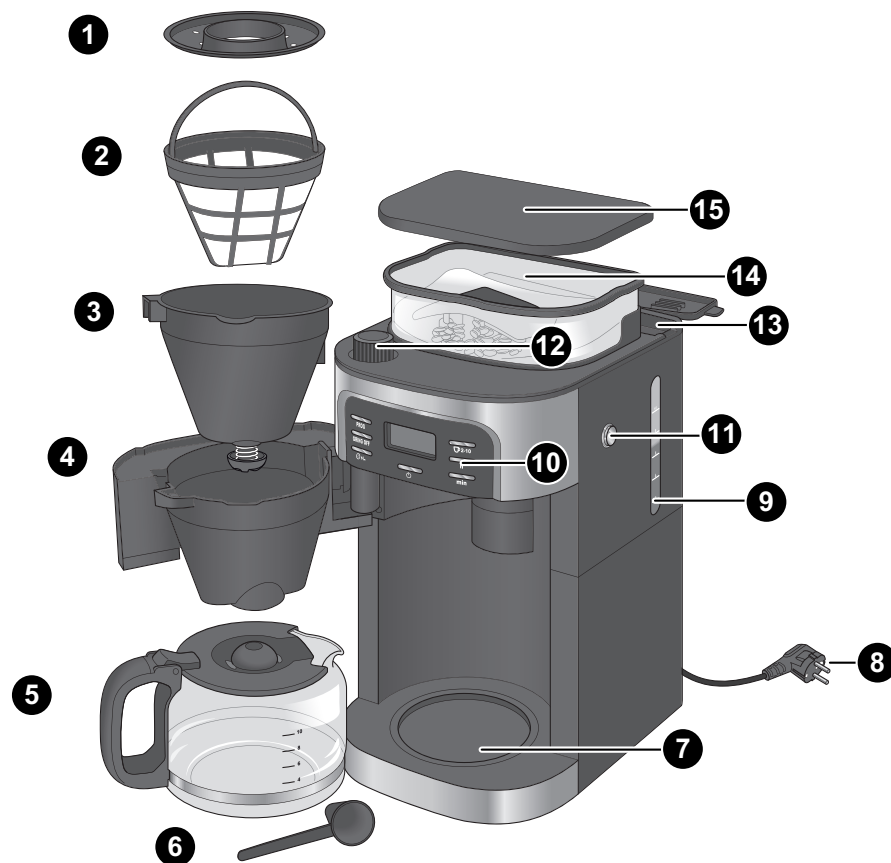
Fig. 1: Parti dell'apparecchio
