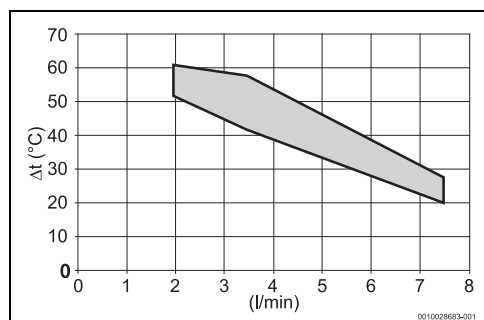
Fig. 31 Modèle 9 litres
