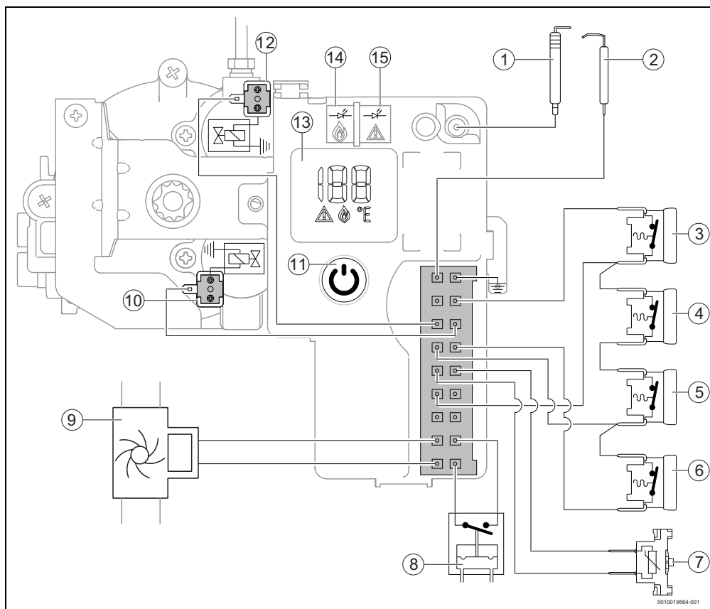
Fig. 30 Schéma de câblage
