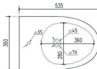
BIDET (art.GIO.41)
