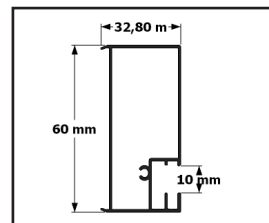
Profil vetro
