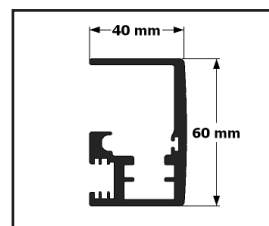
Profilo binario
