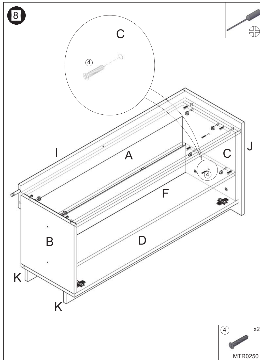
MODULO TV 1P.+1H. "SOKKEL" 104x50 cm.
