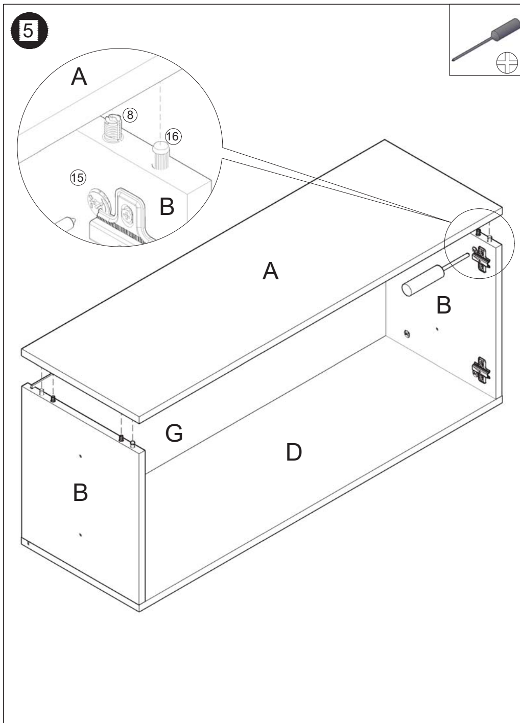
MODULO TV 2P. "SOKKEL" 104x50 cm.
