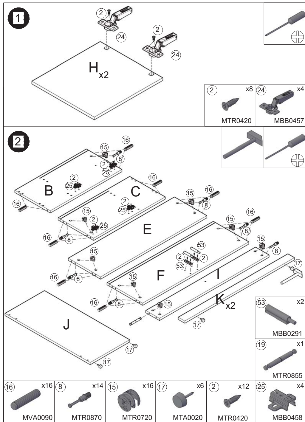
APARADOR 2P. "SOKKEL" 104x80 cm.
